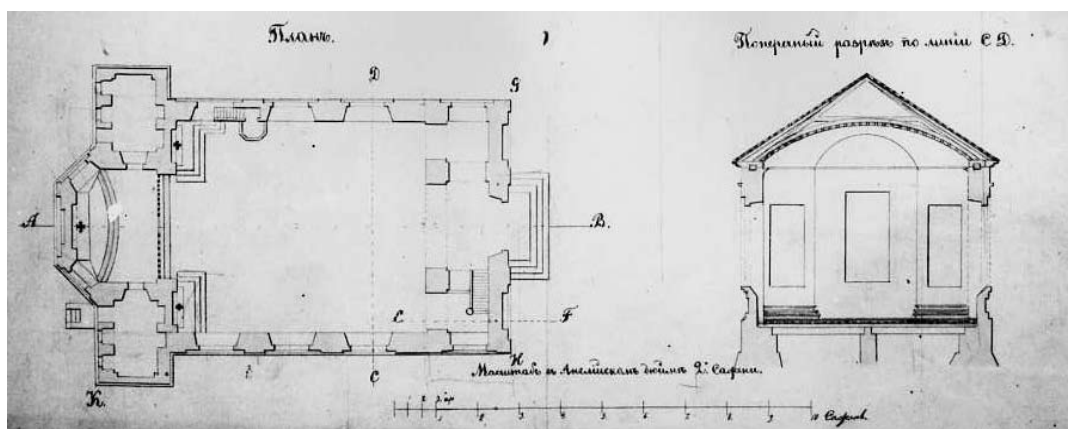
2b. Rzut poziomy kościoła i przekrój poprzeczny wzdłuż linii CD. Центральный государственный архив, S. Petersburg, фонд 218, opis 3, дело 1660, k. 11.
