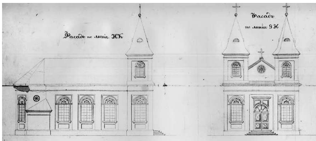
2a. Wygląd zewnętrzny kościoła (projekt). Центральный государственный архив, S. Petersburg, фонд 218, opis 3, дело 1660, k. 11
